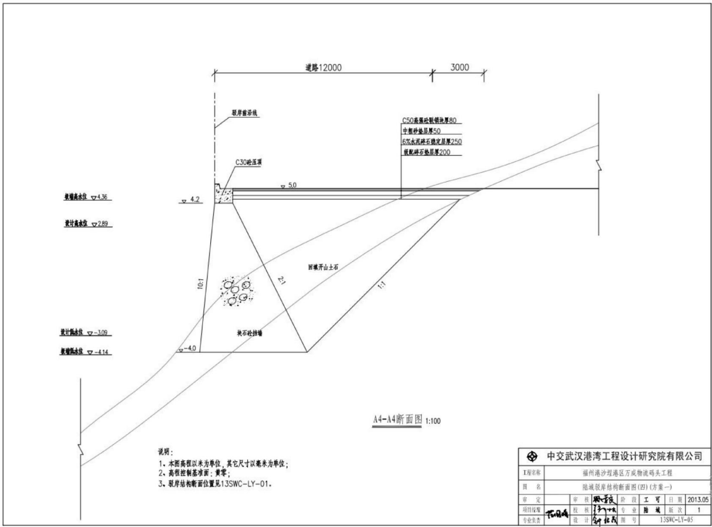
图 2.5-5 项目陆域驳岸结构断面图 (4)
