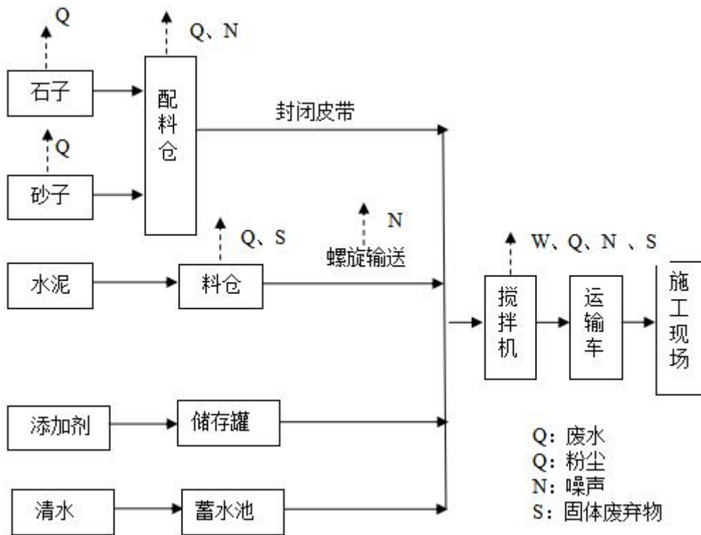
图 2.8-4 搅拌生产工艺流程图
