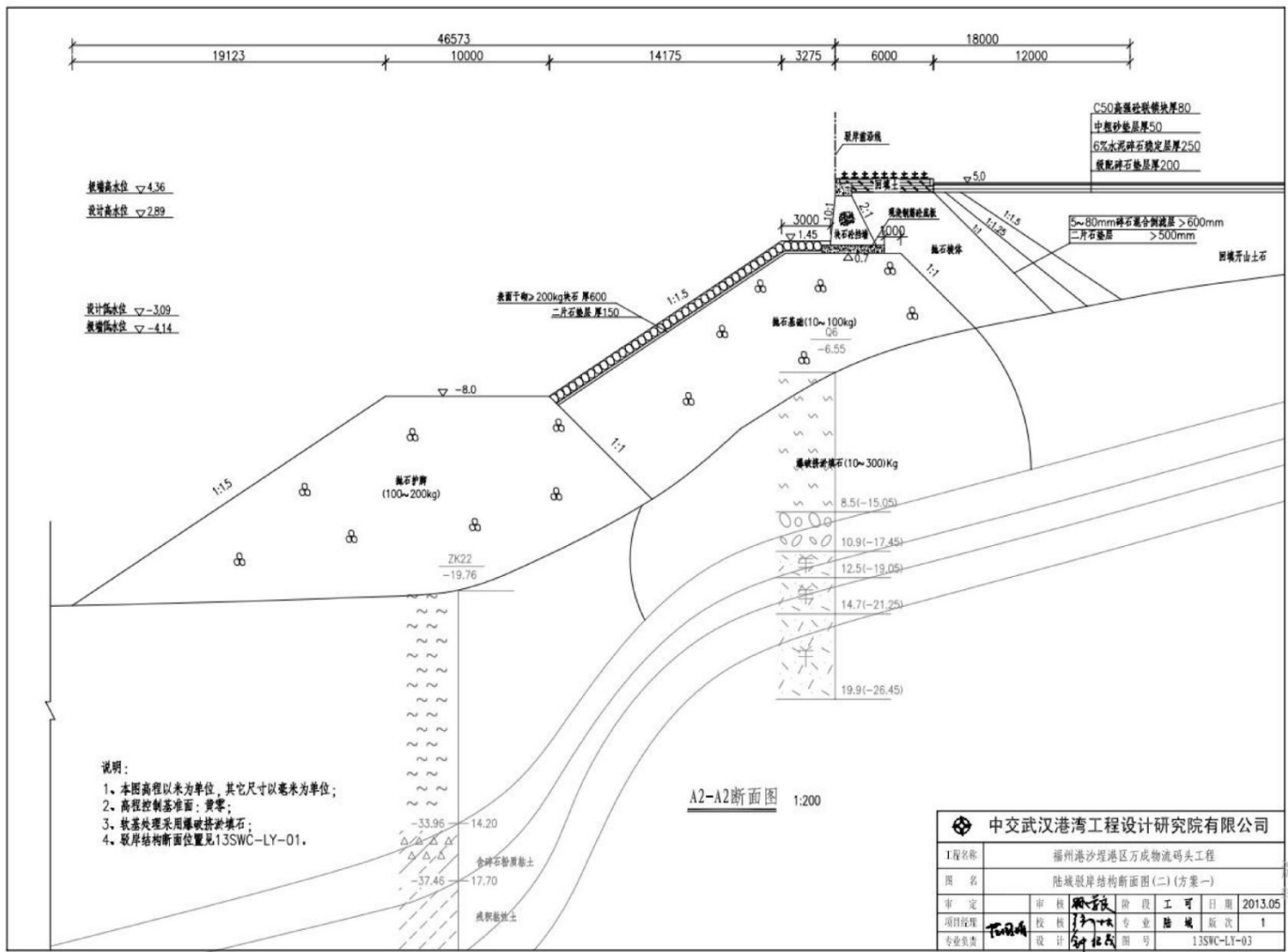
图 2.5-3 项目陆域驳岸结构断面图 (2)
