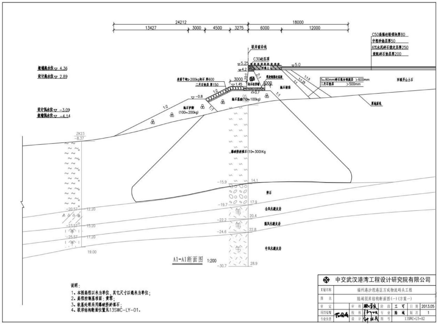
图 2.5-2 项目陆域驳岸结构断面图 (1)
