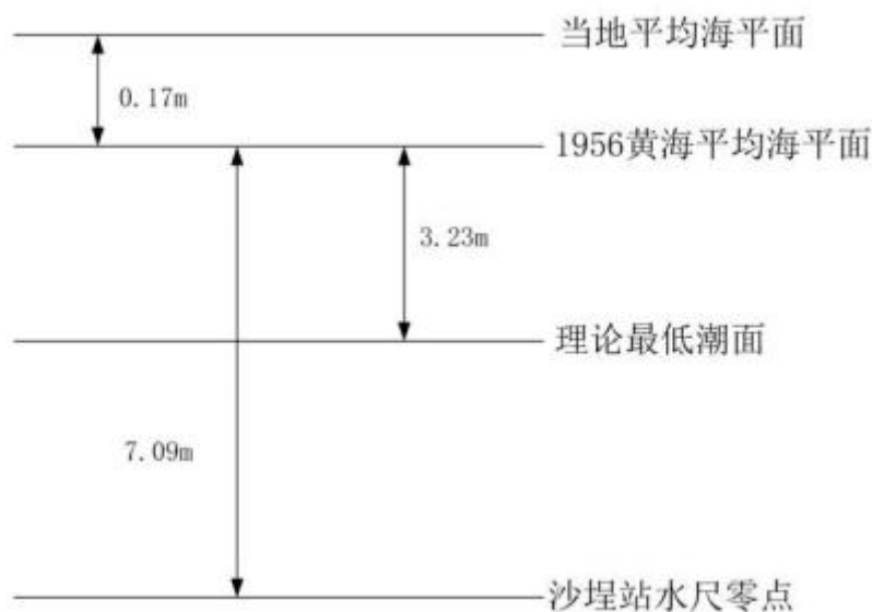
图4.1-1基准面关系
