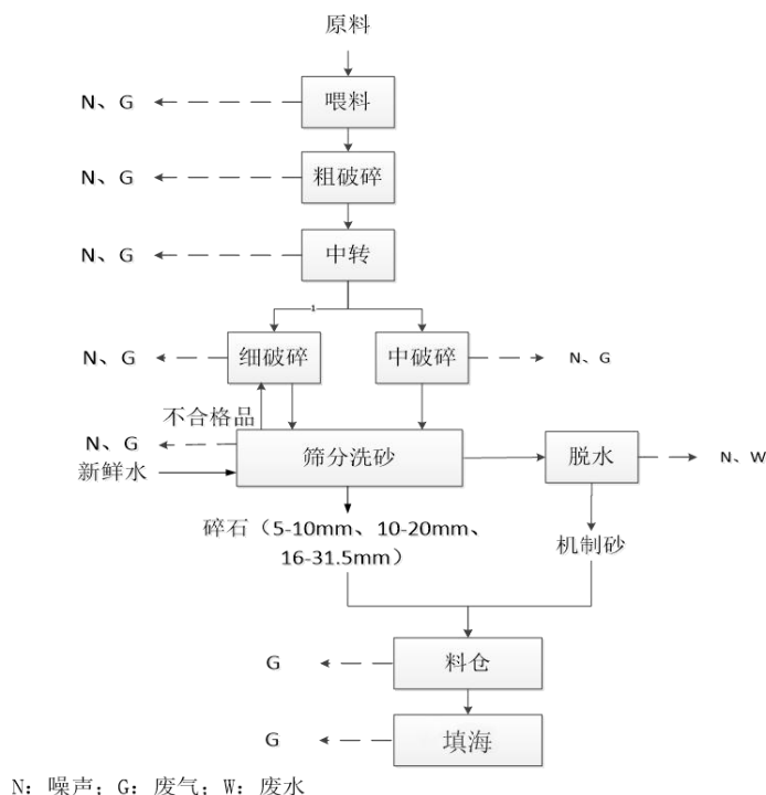
图 2.8-3 加工工艺流程图
