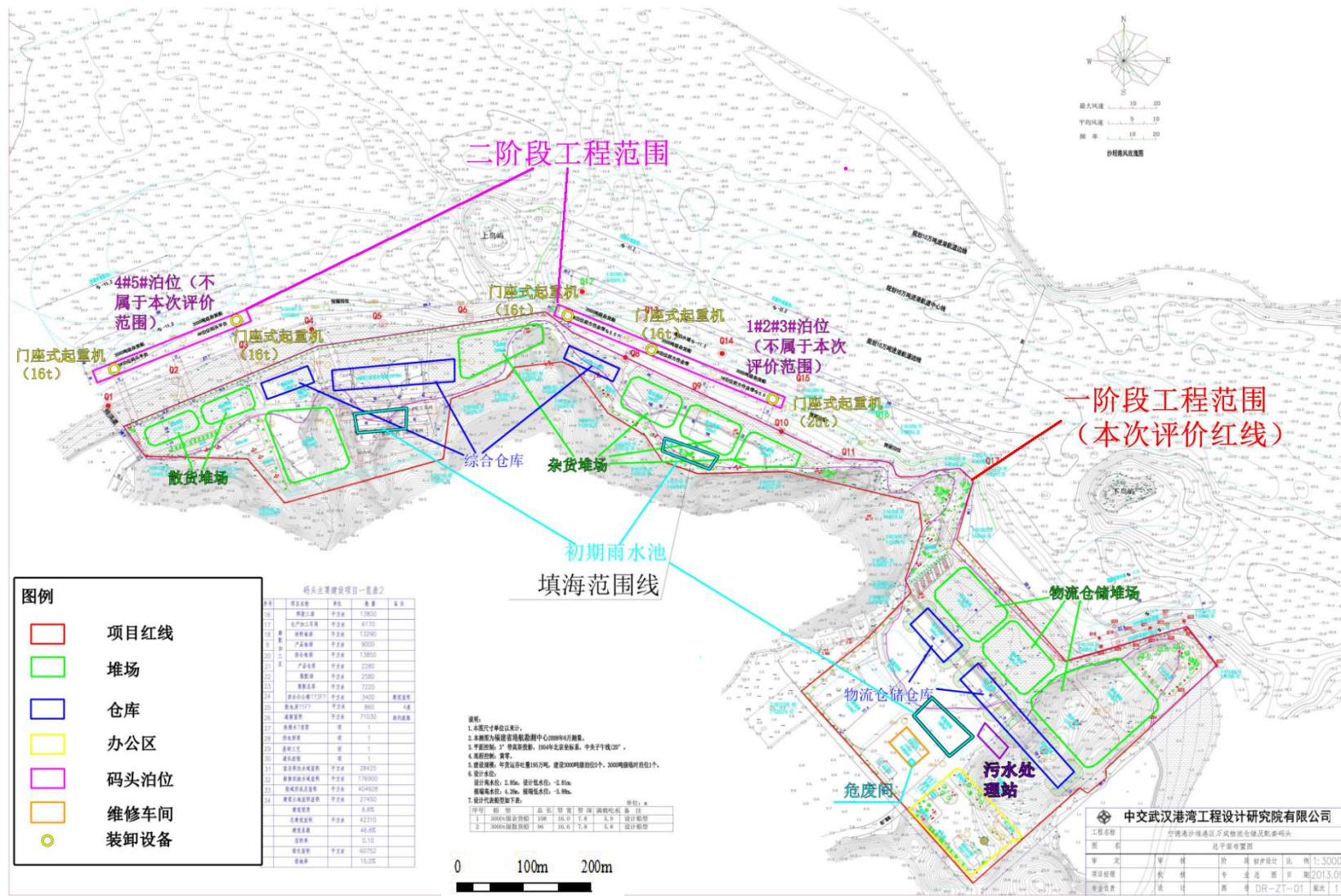
图 2.4-1 项目总平面布置图
