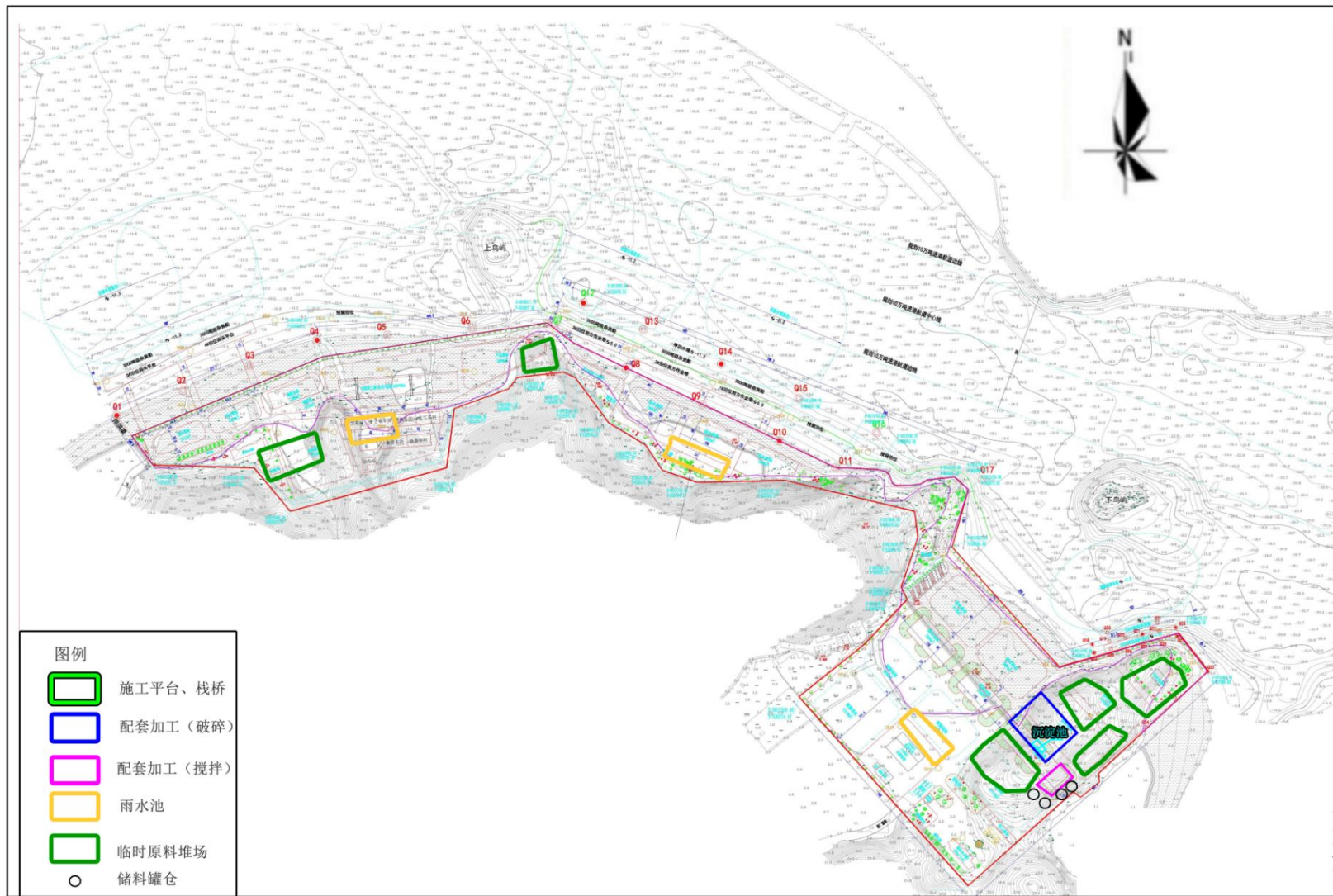
图 2.7-1 施工平面布置图（码头施工不在本次评价范围内）
