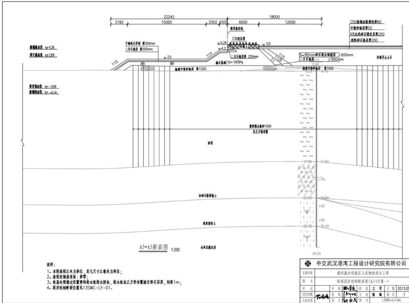
图 2.5-6 项目陆域驳岸结构断面图 (5)
