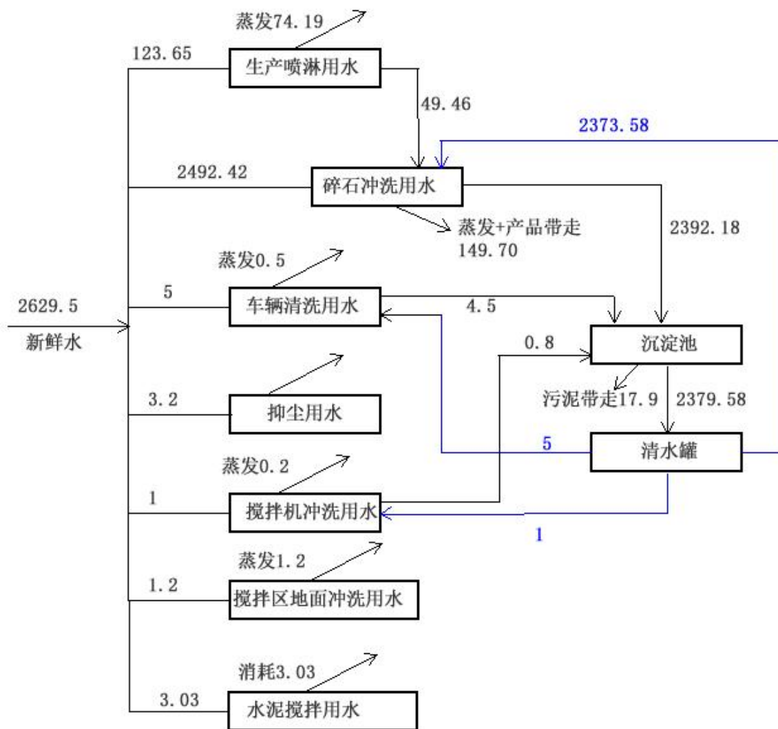
图 3.1-1 配套加工区最大日水平衡示意图 单位: t/d
