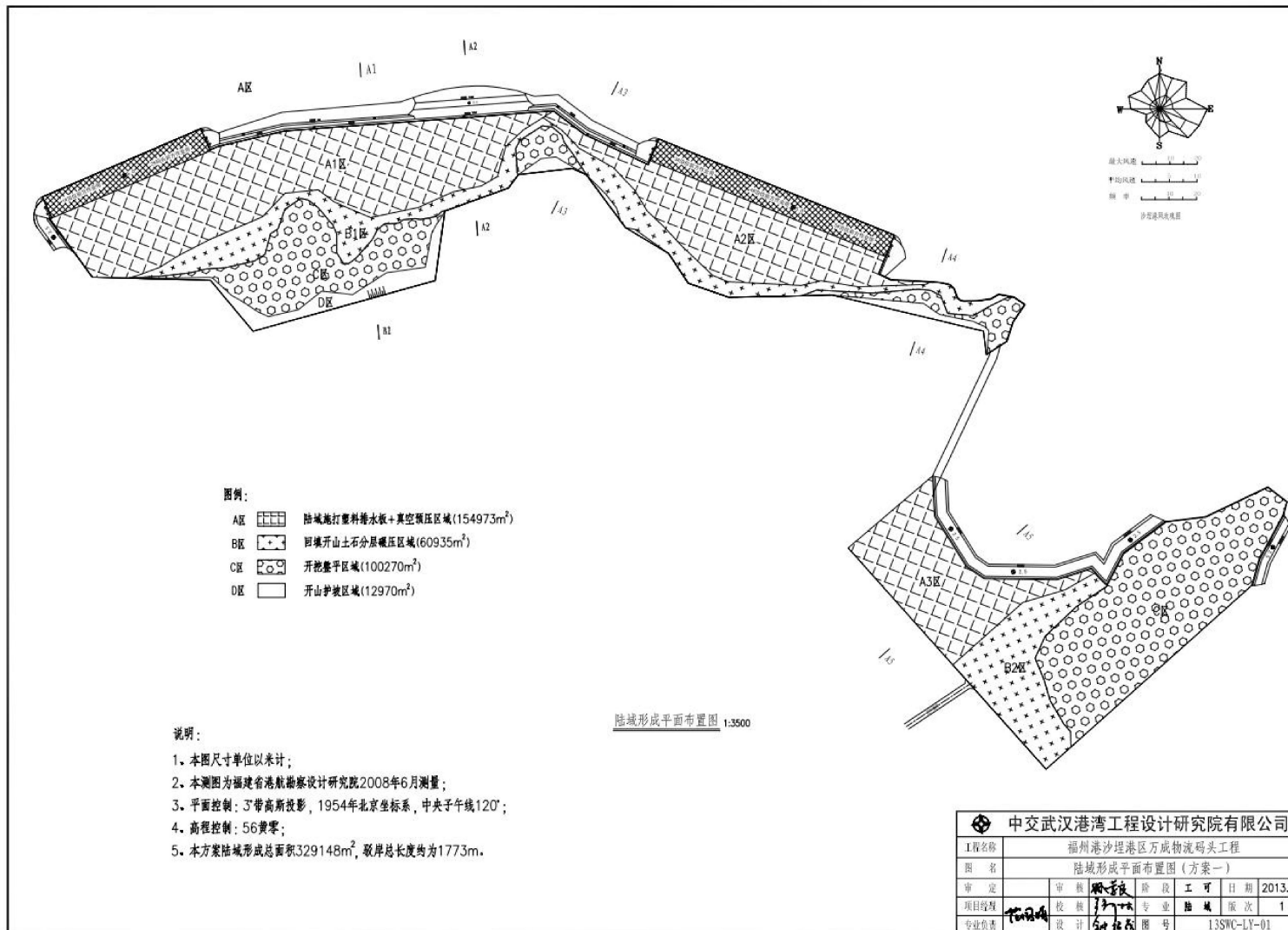
图 2.5-1 项目陆域形成平面图
