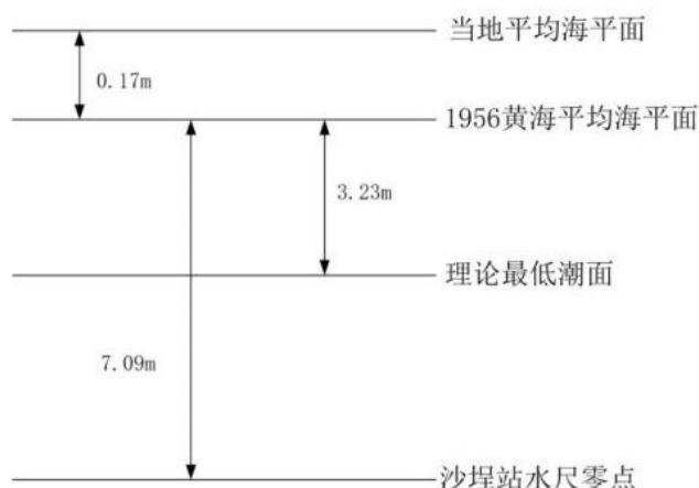
图 5.1-1 基准面关系图
