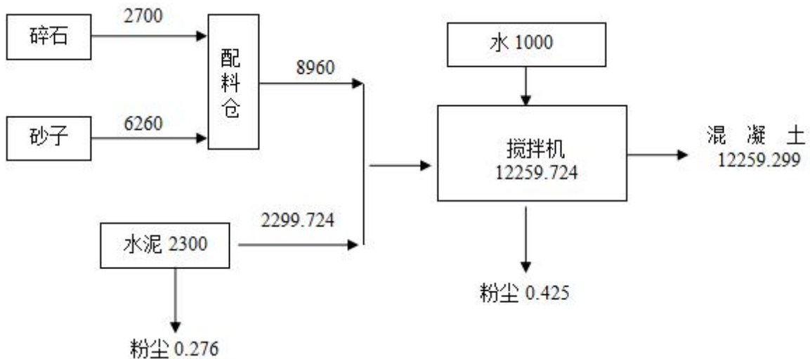
图 2.8-5 混凝土生产物料平衡图（单位：t/a）
